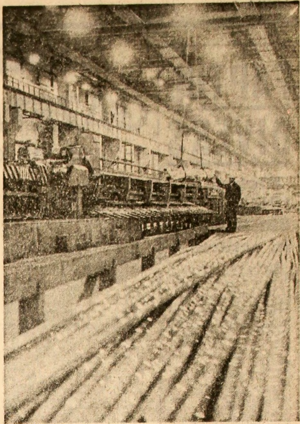
Uzina de prelucrare a aluminiului din Slatina. Colectivul său de muncă și-a depășit substanțial sarcinile de plan, asimilând, totodată, zeci de noi sursoare intens solicitate de economie. In imagine: secția metalurgică I a uzinei. Foto: E. Dichisescu
