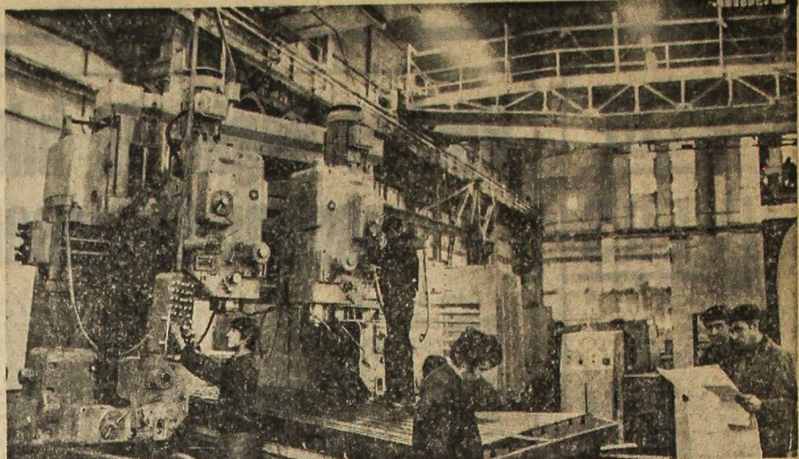
La Întreprinderea „23 August” din București se instalează noi mașini și utilaje care vor mări capacitatea de producție a secțiilor de prelucrare mecanică. În fotografie: echipa condusă de Dumitru Joca reglînd o mașină de frezat
