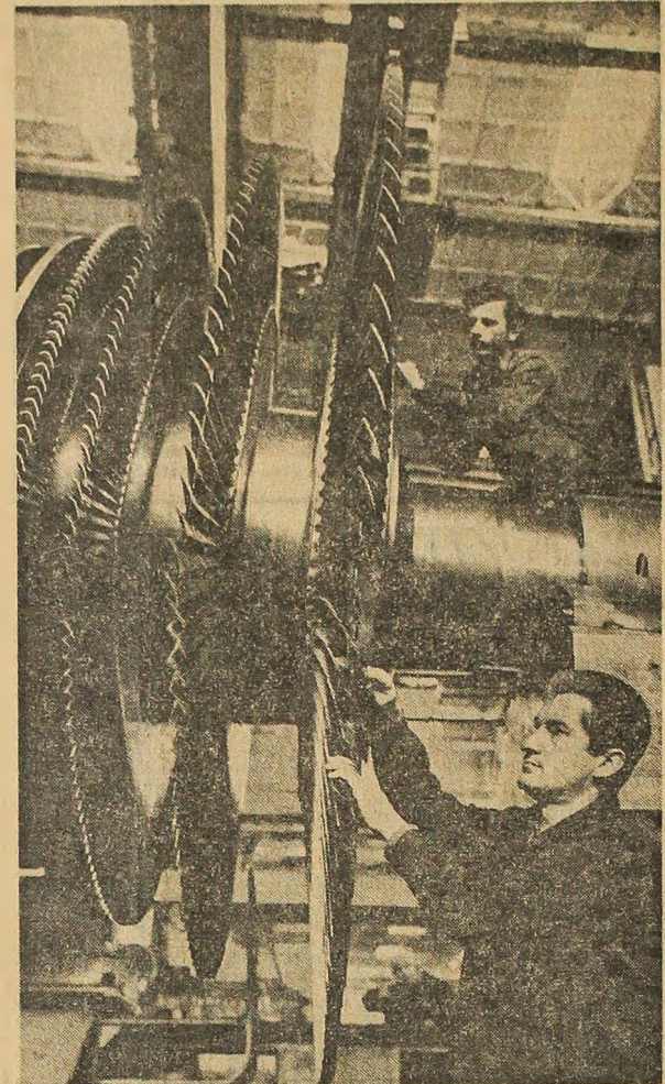
La întreprinderea de mașini grele din București se verifică peletele rotorului pentru turbinele cu o putere de 330 MW
