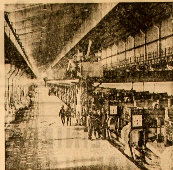
Uzina de aluminiu Sîlîna. Aspect din noua hală de electroliză
