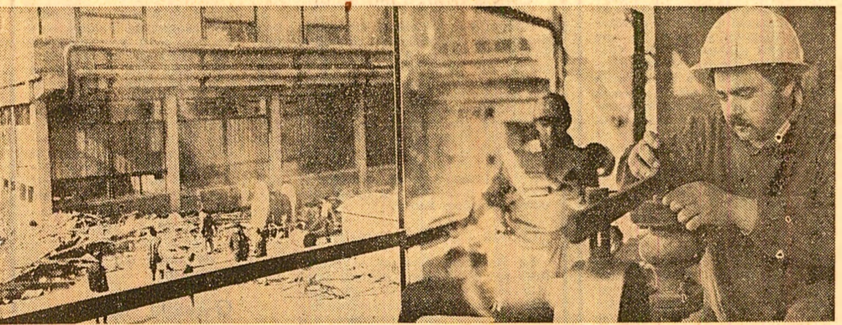
O lucrare deosebită în centrul atenției generale pe șantierul întreprinderii „Timpuși noi” — centrala termoelectrică; montajul cazanului de apă fierbinte, la care lucrează lăcătușul Alexandru Soare și sudorul Ion Hincu
