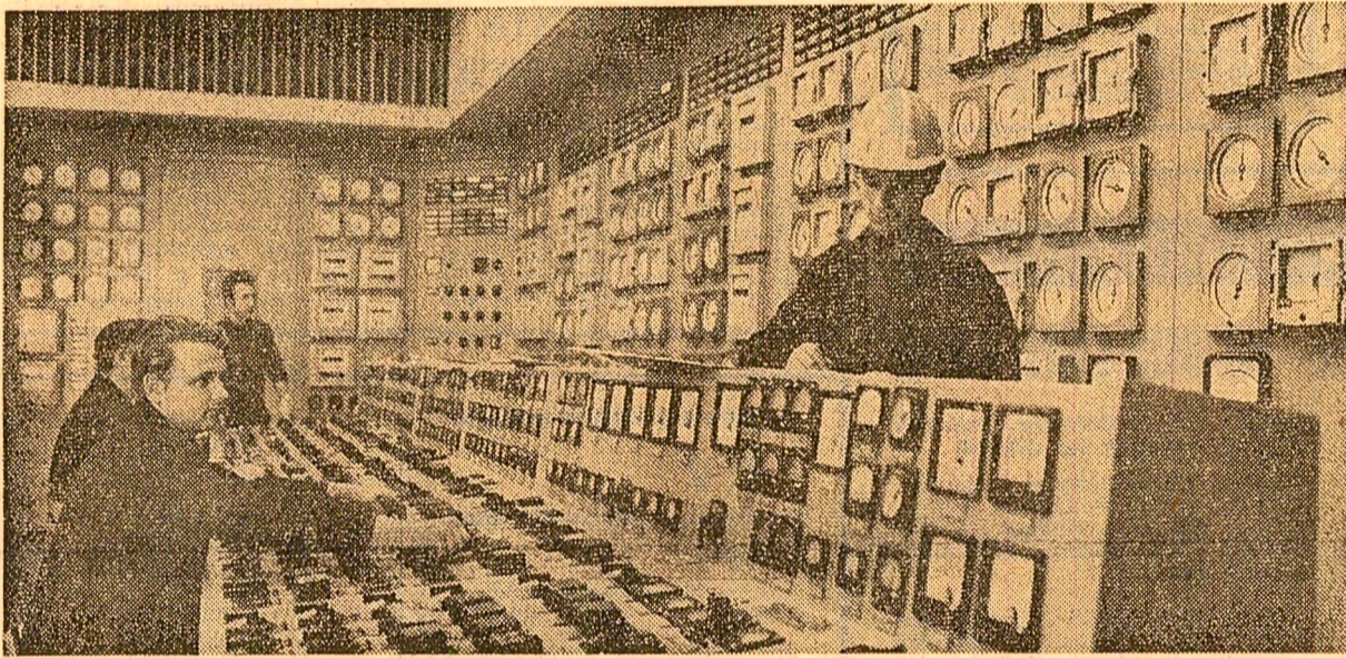
Termocentrala Mintia-Deva, creația a acestui cincinal, în care — alături de creșterea producției de energie electrică — se obțin importante economii de combustibili. În imagine: tabloul central de comandă a agregatelor energetice ale termocentralei
