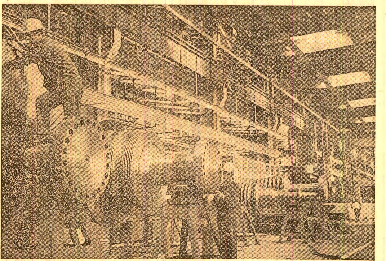
Întreprinderea de mașini grele din București: se lucrează la ansamblarea unei noi turbine de 330 MW Foto: E. Dichiseanu
