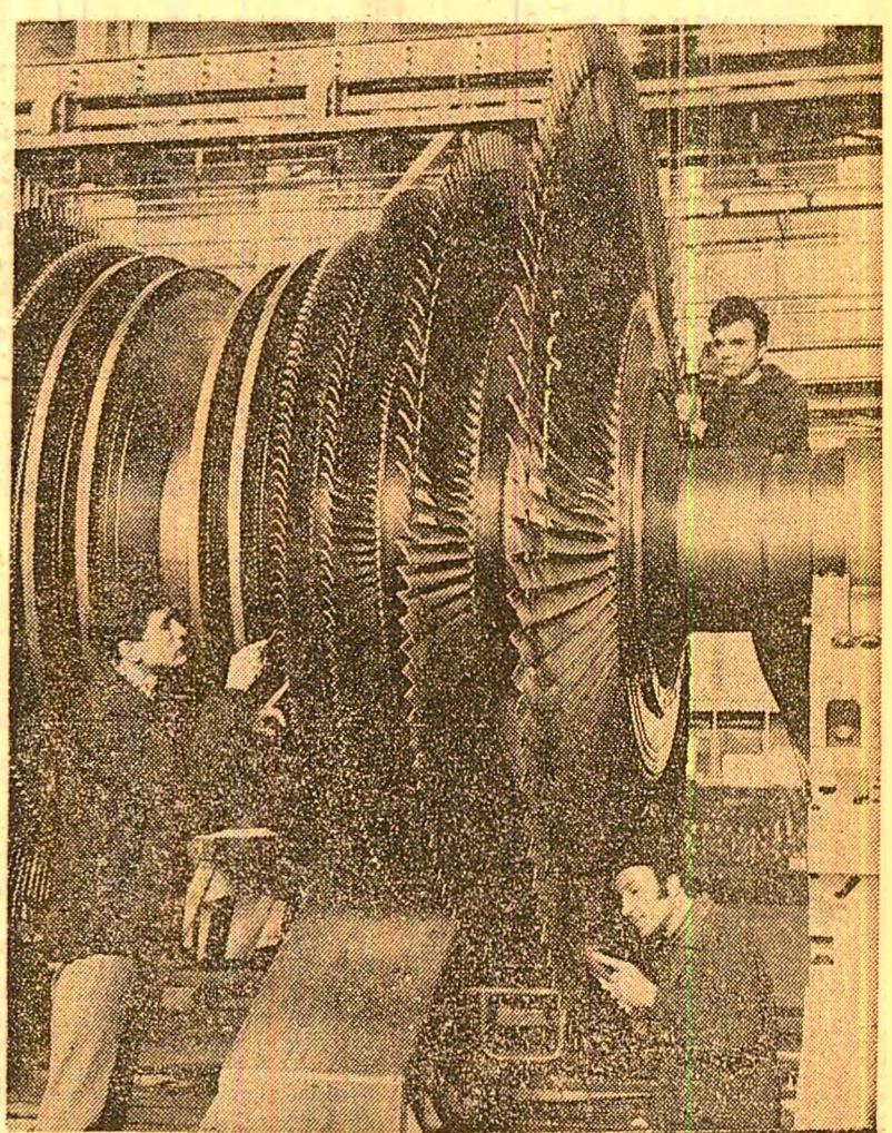
Intreprinderea de mașini grele din Capitală: ultimele finisări la rotorul unei turbine de mare capacitate
