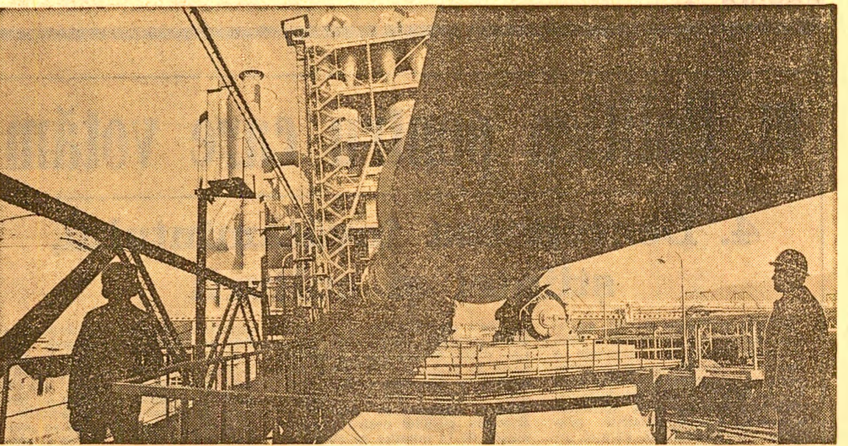
Fabrica de ciment din Fieni — județul Dimbovița. În imagine: noua linie tehnologică cu o capacitate de 3000 tone ciment în 24 de ore, realizare de prestigiu a industriei noastre constructoare de mașini. Foto: S. Cristian
