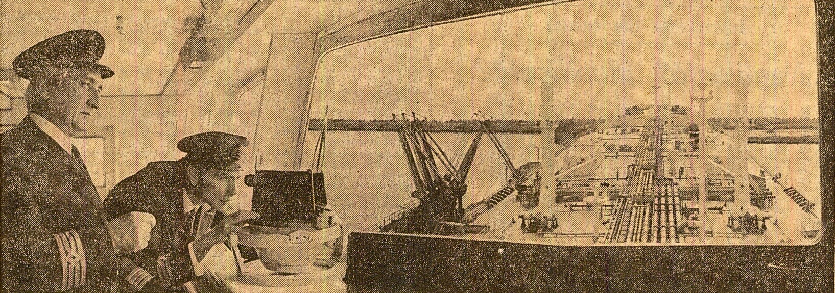
La puntea de comandă a navei „Banatul” — de 86 000 tdn — intrată recent în dotarea flotei românești; în prim plan, comandantul navei, Gheorghe Ungureanu, și secundul Nicolai Cristian-Cosma. Foto: S. Cristian
