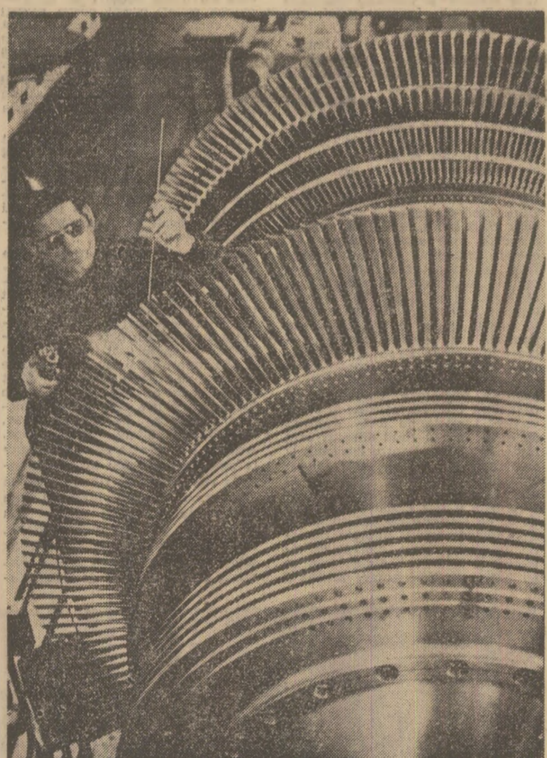
La I.M.G. București a căpătat contur rotorul unei noi turbine de 330 MW
