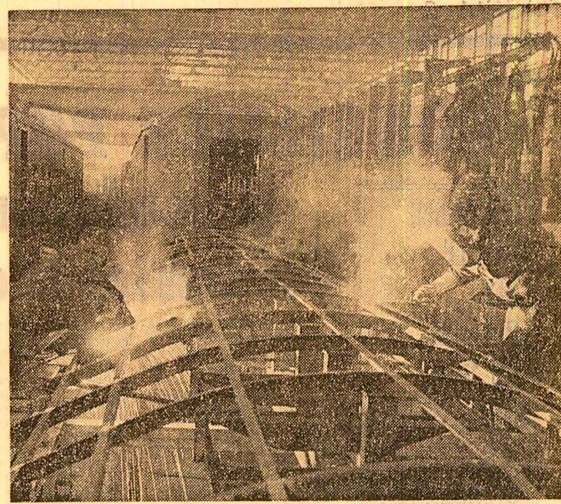
Întreprinderea de vagoane din Arad: prinde contur un nou vagon de călători
