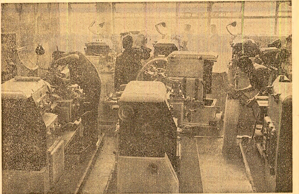
Se montează noi tipuri de strunguri la întreprinderea de strunguri din Arad, al cărei colectiv — în acest an — este puternic angajat în înnoirea și modernizarea producției
