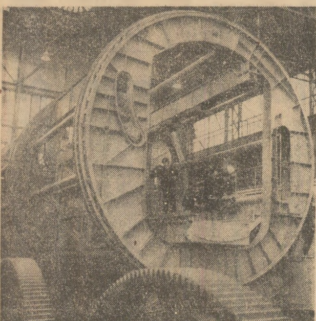
Culbutor de vagoane (mecanism de răsturnare a vagoanelor) — piesă destinată exportului, executată în secția mecanică grea a uzinelor „23 August“ din Capitală
