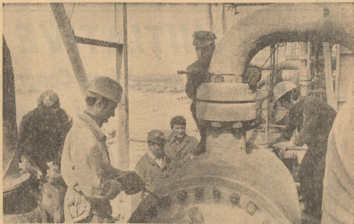
La Combinatul chimic din Turnu Măgurele se execută ultimele lucrări de reparații la un important agregat Foto: S. Cristian
