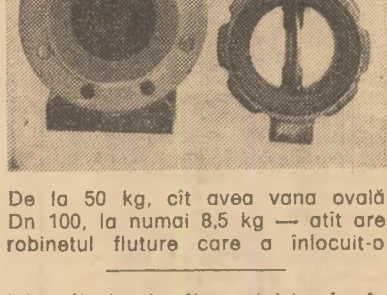
De la 50 kg, oit avea vana ovală Dn 100, la numai 8,5 kg — oit are robinetul fluture care a înlocuit-o.
