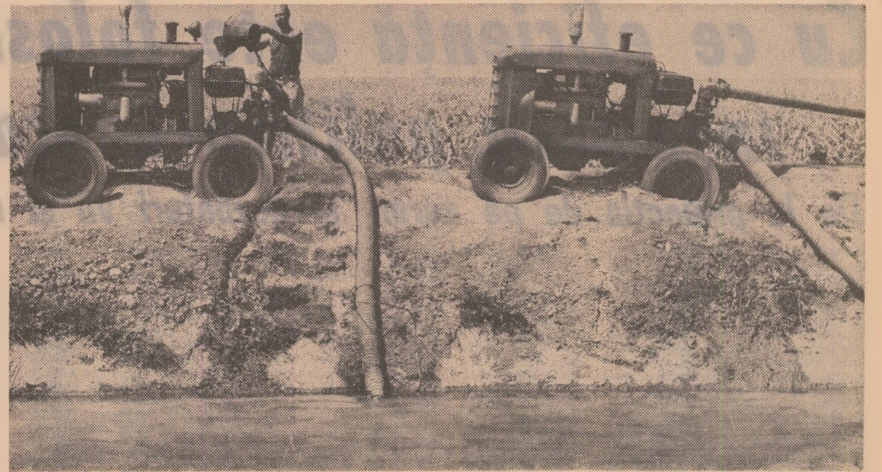
Cele două motopompe de la C.A.P. Ștefan Vodă, județul Ialomița, supravegheate în permanență de mecanicul Marin S. Dumitru, trimis în lanuri apă necesară culturilor
