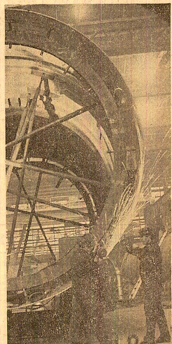
La întreprinderea „Grivița roșie“ din Capitală se acordă o atenție deosebită realizării unor produse de înalt nivel tehnic și calitativ. La unul dintre asemenea produse se lucrează în prezent la secția cazangerie, de unde prezentăm imaginea alăturată.
