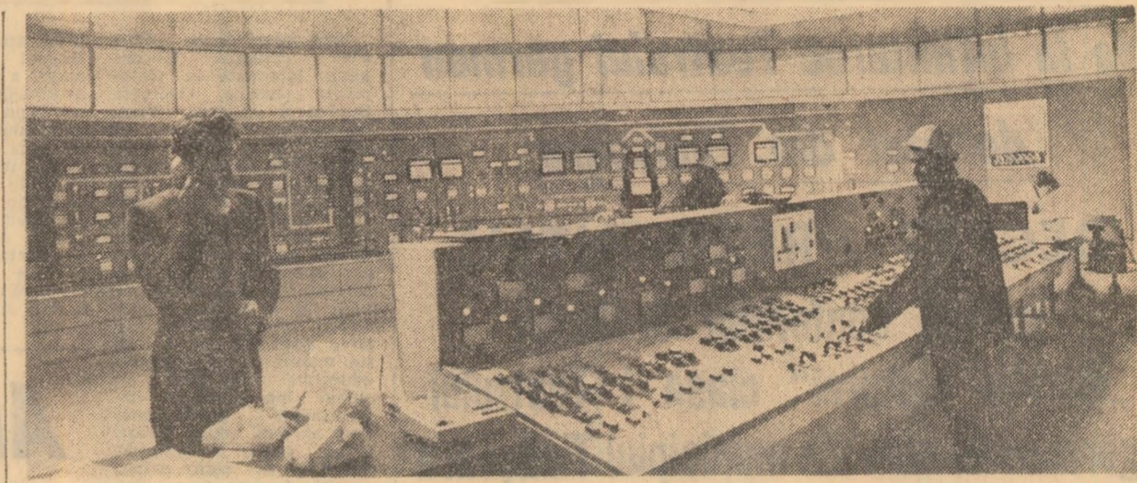
Furnalul „amiral“ al siderurgiei românești, așa cum a fost denumit furnalul nr. 5 de la Combinatul siderurgic Galați, recent pus în funcțiune, impresionează oțit prin dimensiunile sale, cit și prin înalțul grad de tehnicitate și automatizare al instalațiilor
