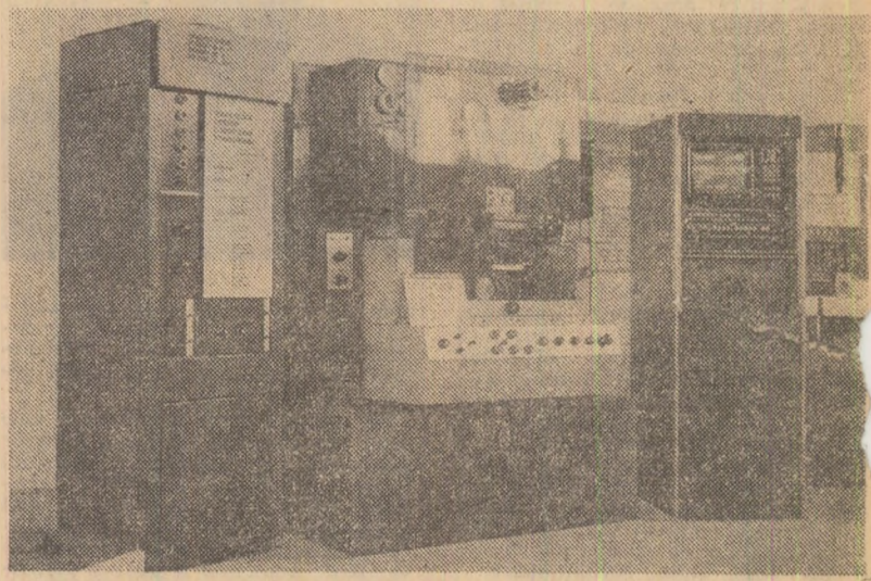
NUMEROM CNC-450 AC, ataşat unei maşini de prelucrare prin electroeroziune cu fir
