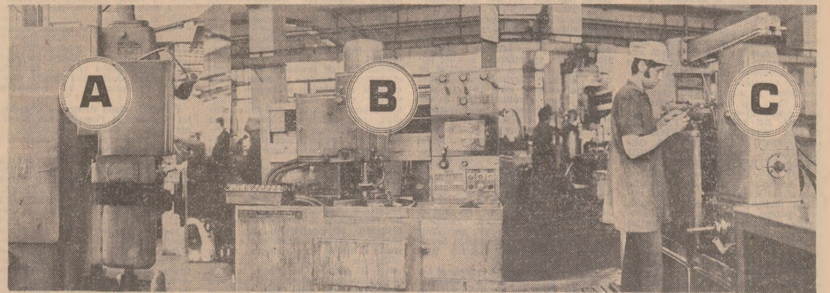
POLIDESERVIRE = POLICALIFICARE. O condiție pentru extinderea polideservirii este policalificarea. În imagine, muncitorul Adrian Voicu, care lucrează simultan la 3 utilaje diferite: A) mașina de șevăruit; B) mașina de danturat prin mortezare; C) mașina de danturat prin frezare.
