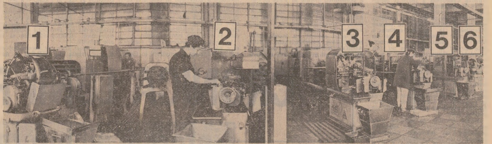
UN MUNCITOR DE ÎNALTĂ CALIFICARE LUCREAZĂ LA 6 MAȘINI. Organizându-se munca pe baza unei ciclograme a folosirii timpului, regiului Florian Buligă (în fotografie) lucrează, ajutat de Cristian Jinga, muncitor cu categoria a II-a, simultan la 6 strunguri automate monoax, în condițiile în care ciclul de prelucrare a unei piese nu depășește un minut.
