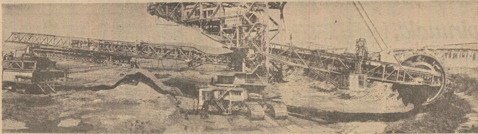
Utilaje de înaltă tehnicitate în carierele de extracție a cărbunelui din bazinul Gorjului.
