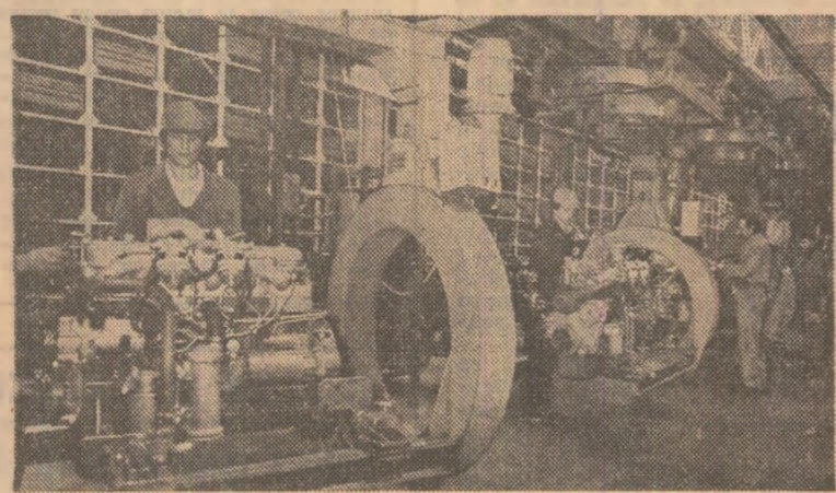
Linia de montaj al motoarelor diesel a Întreprinderii de autocamioane Brașov
