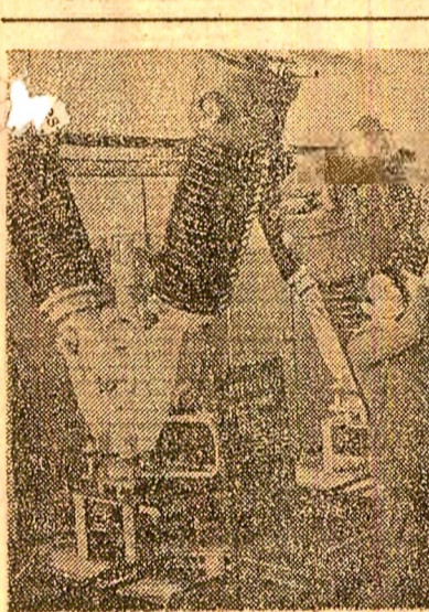
Întreprinderea „Electroputere” din Craiova: se efectuează probele de funcționare la un nou lot de interupătoare de înaltă tensiune
