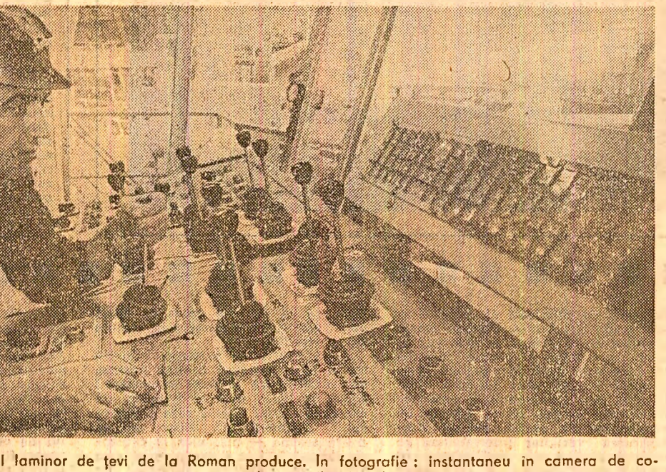
Noul laminor de țevi de la Roman produce, în fotografie: instantaneu în camera de comandă a noilor instalații. Foto: S. Cristian
