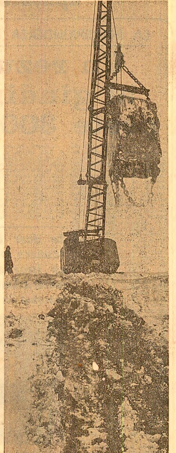
La Platca, canalul magistral de aducțiune a apei în sistemul de irigații Vîșoara este curățat de mil cu utilaje de mare capacitate
