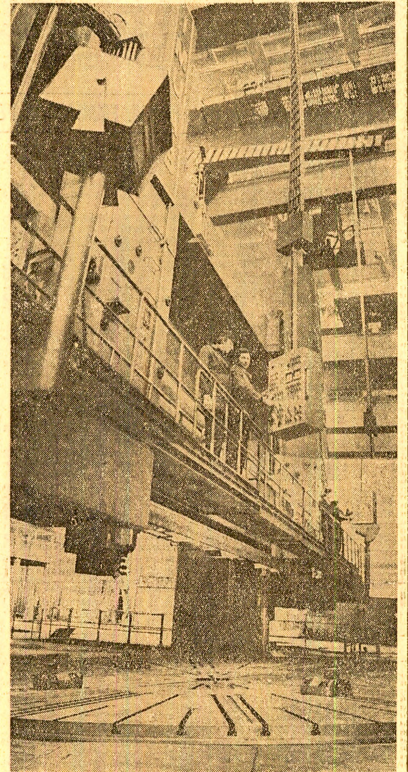
Strungul carusel cu diametrul de 16 000 mm — o remarcabilă creație a științei și tehnicii românești. Construit în cunoscuta Întreprindere de mașini-unelte și agregate din Capitală, la realizarea lui au colaborat 9 institute de cercetare științifică și de învățământ superior și 28 de unități industriale din țară, sub coordonarea proiectantului general — Institutul de cercetare științifică și inginerie tehnologică pentru mașini-unelte „Titan” din București
