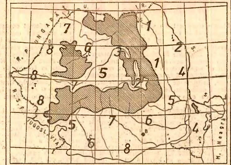
Temperatura solului (în grade Celsius) la 10 cm adâncime (30.03.1985)
