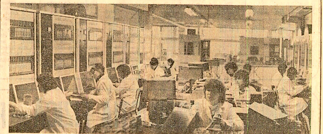
Ca urmare a muncii bine organizate, a eforturilor făcute în ultima perioadă, colectivul întreprinderii „Electrotehnică” din Capitală și-a realizat și-a depășit planul la export pe primul trimestru al acestui an. În fotografie: standul de reglare și testare a blocurilor electronice, unde se face o ultimă verificare a calității echipamentelor electronice destinate exportului
