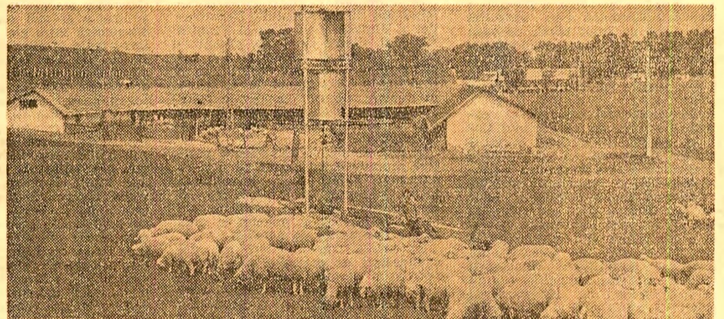
Cu ajutorul energiei vîntului, această instalație pompează apa necesară pentru tabăra de vară — ovine a C.A.P. Fălcui, județul Olt
