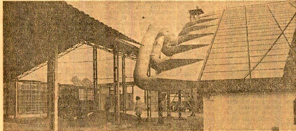
La Oltenița se află în funcțiune această instalație cu captatoare solare pentru uscarea cerealelor
