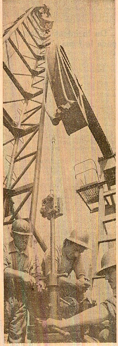
La realizarea producției de țiței, un rol de mare însemnătate îl au brigăzile de intervenții, chemate să repare sondele în funcțiune cu maximum operativitate. În fotografie: brigada de intervenții condusă de Victor Avădanei, de la schelele Clejani. Foto: Sandu Cristian
