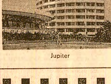
Jupiter
