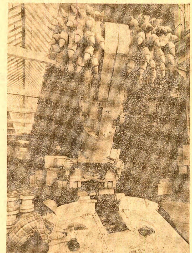
La Intreprinderea mecanică Timisoara se produce o gamă largă de utilaje miniere destinate bazinelor carbonifere.
