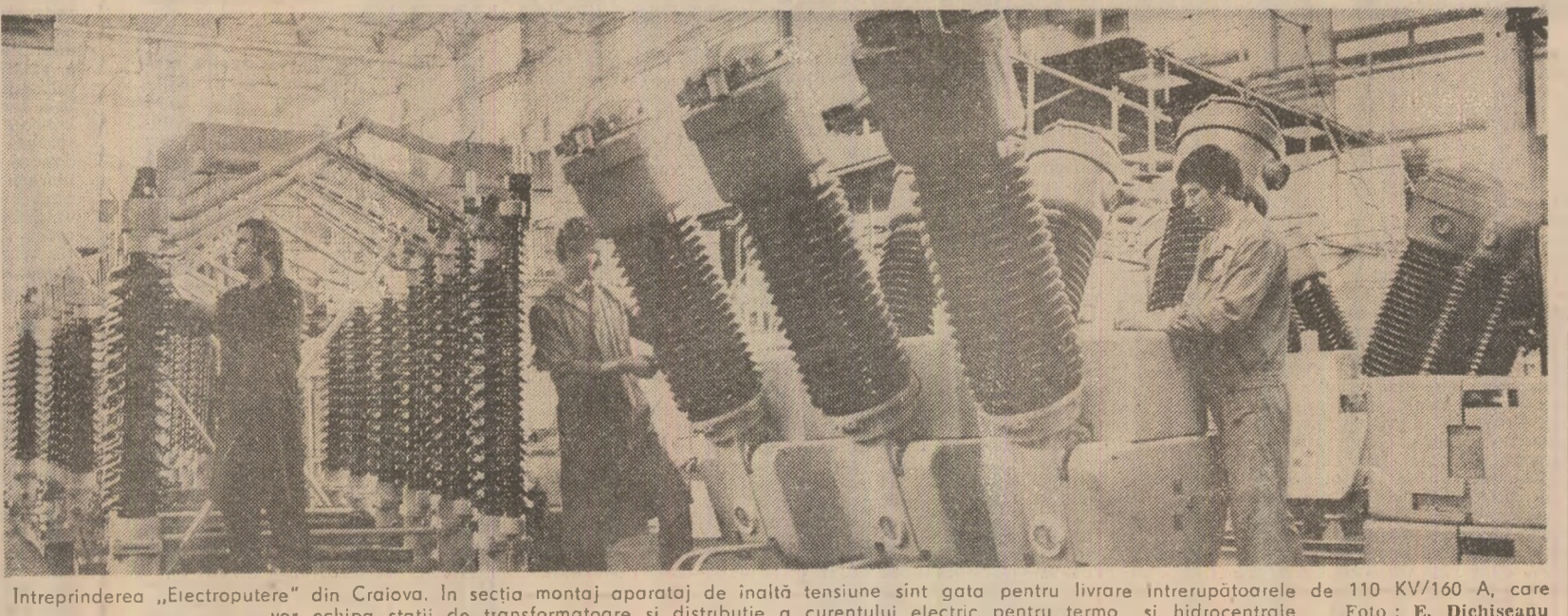
Întreprinderea „Electroputer” din Craiova. În secția montaj aparatelor de înaltă tensiune sînt gata pentru livrare intrerupătoarele de 110 KV/160 A, care vor echipa stații de transformatoare și distribuție a curentului electric pentru termo și hidrocentrale. Foto: E. Dichiseanu
