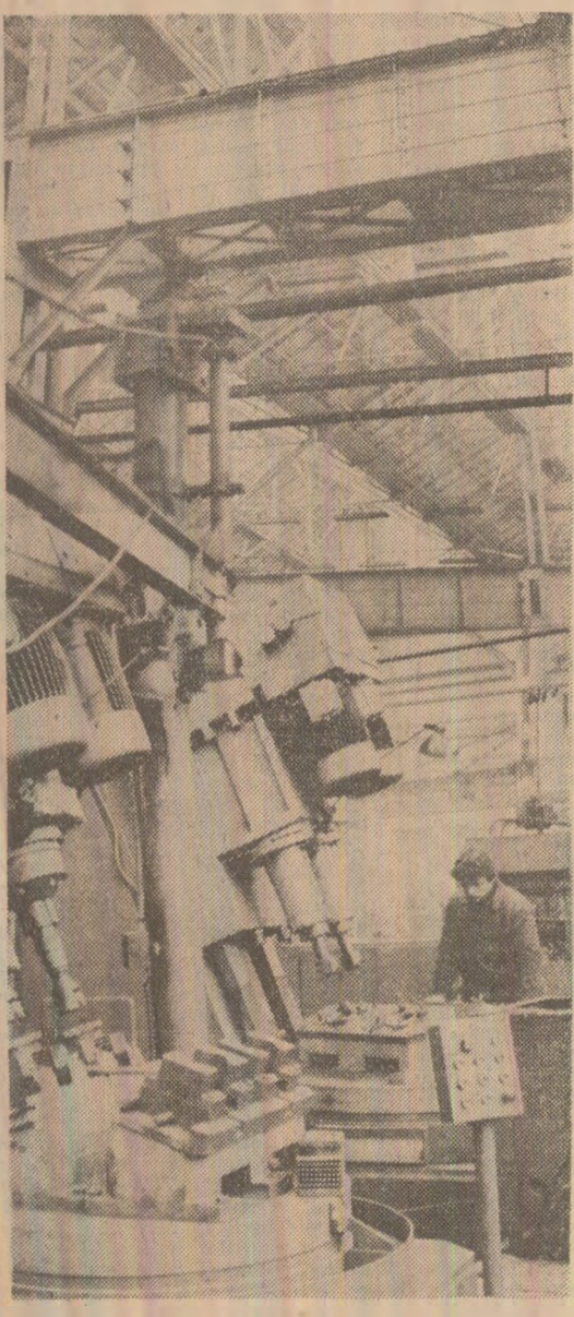
Întreprinderea „Timpuri noi”, din Capitală. În secția prelucrării mecanice, mașini și utilaje, care lucrează în regim automat, sînt prelucrate piese și subansamble necesare motocompresoarelor de mare putere, asimilate recent în fabricația de serie. Foto: E. Dichiseanu
