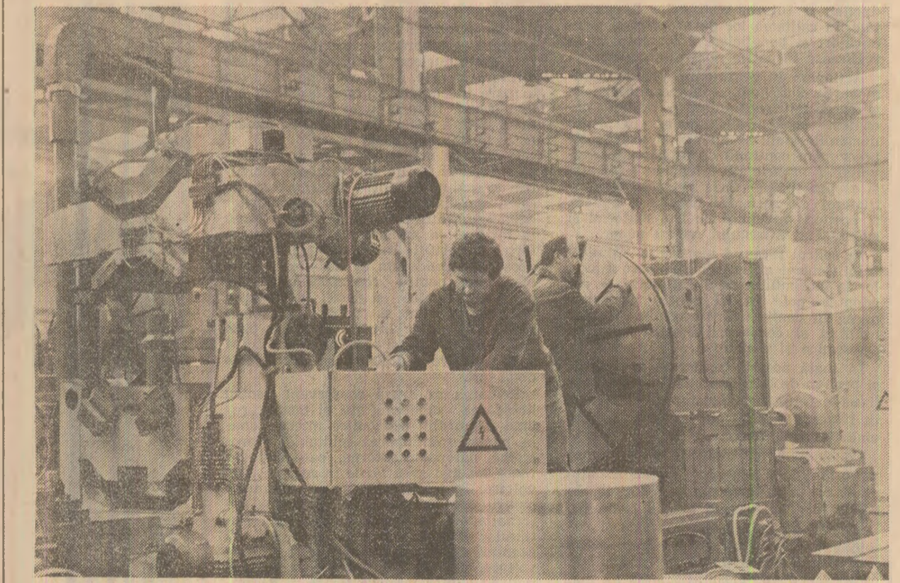
Întreprinderea de mașini-unelte din Suceava: în secția de montaj strunguri Foto: Eugen Dichiseanu
