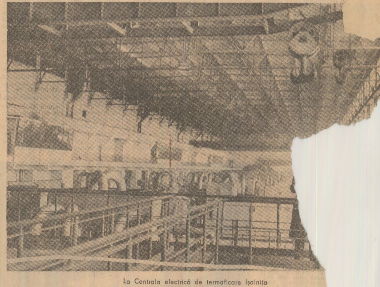
La Centrala electrică de termoficare Ișalnița
