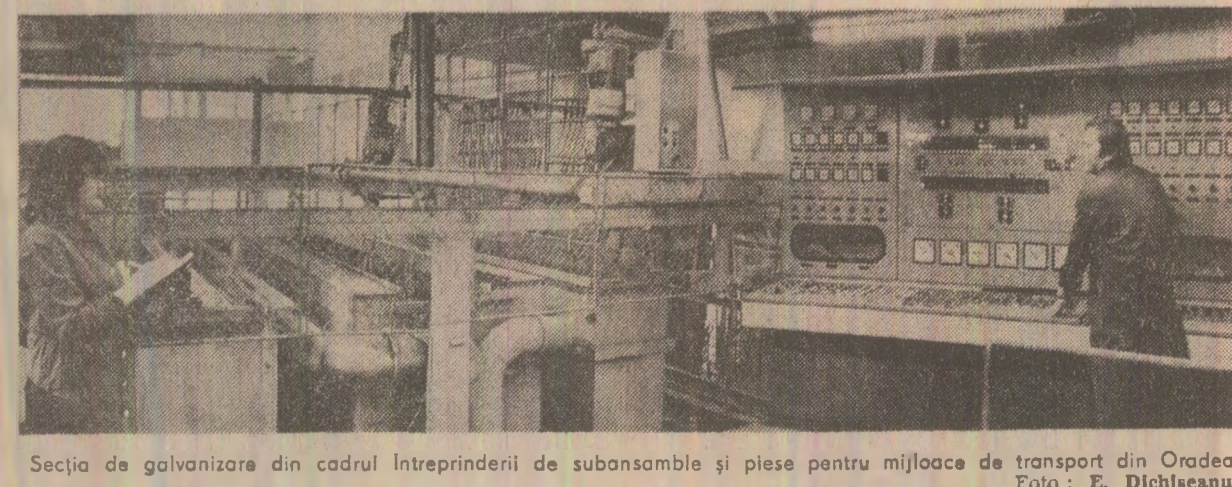
Secția de galvanizare din cadrul întreprinderii de subsansamble și piese pentru mijloace de transport din Oradea Foto: E. Dichisaeau
