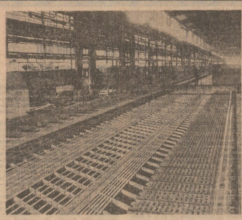
Laminorul de profile mici de la Combinatul siderurgic Hunedoara
