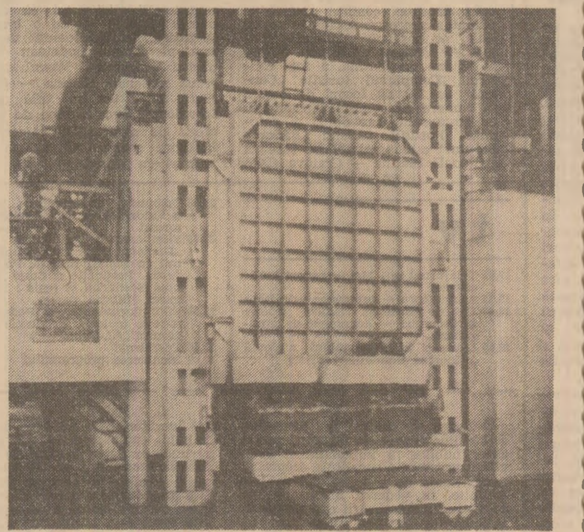
Unul din cuptoarele de forj de la Intreprinderea de Mașini Grele București, la care, prin instalarea arzătoarelor cu recuperare regenerativă de energie, se obțin însemnate economii de gaz metan
