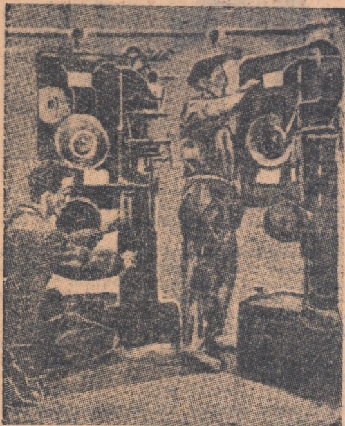
Fabrica „Arta textilă”, din Timișoara, construiește aparate de laborator pentru industria textilă. Muncitorii Al. Gyémánt și Vladimir Lengvardschi montează noi dinamometre (aparate pentru aflarea rezistenței țesăturilor la întindere).
