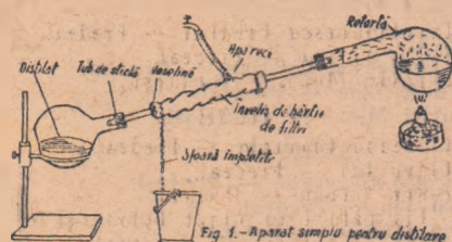
Fig. 1. Aparat simplu pentru distilare
