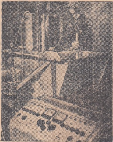
Aparat ultrasonor pentru descoperirea defectelor de fabricație din anvelopele de cauciuc.
