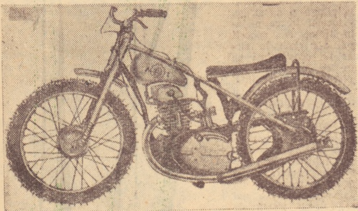
1. O motocicletă sovietică pentru curse pe gheață, realizată prin montarea unui motor de I. J. pe rama motocicletei K.125.
