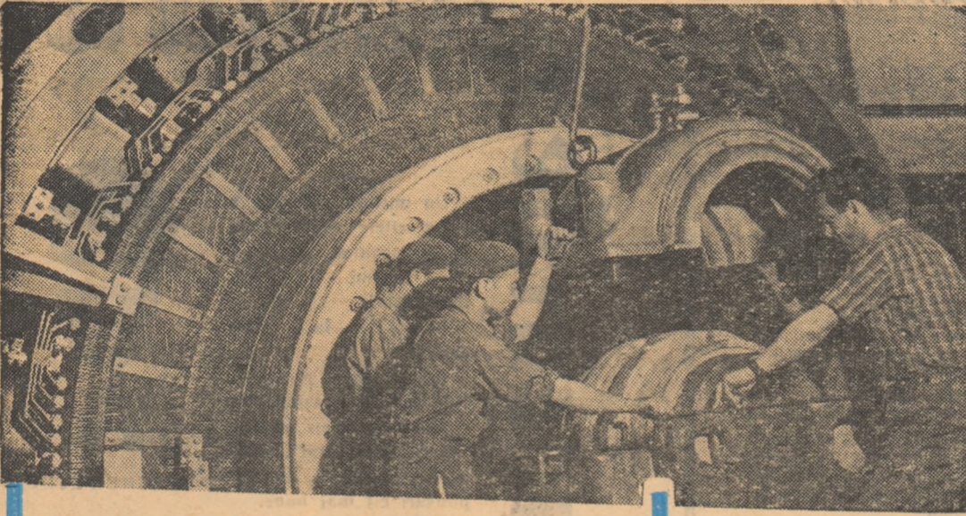
La un deceniu de la naționalizare, Hunedoara a devenit cu adevărat o cetate a oțelului. Aici se va naște în curând un nou gigant: laminorul Blumming. În fotografie, montarea unuia din agregatele laminorului.
