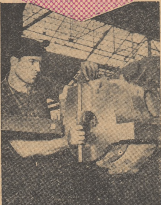
Arborele cotit al motorului S-50 e o piesă voluminoasă, dar și aici trebuie precizie! În fotografie: strungarul Fleagă Petre, de la uzina „Timpuri Noi” din Capitală, verifică exactitatea dimensiunilor.
