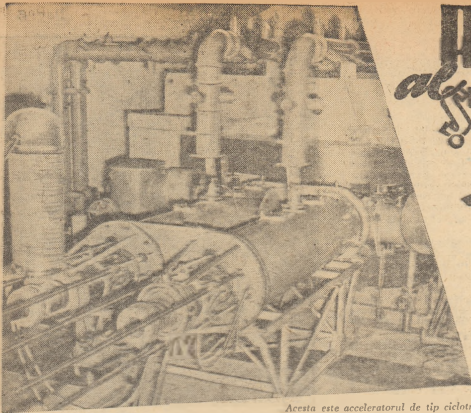
Acesta este acceleratorul de tip ciclotron folosit de cercetătorii de la Institutul de fizică atomică.
