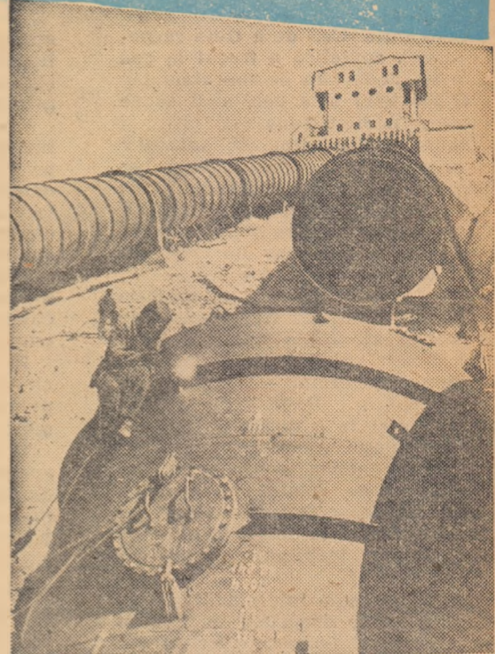
Pe cursul căderii de apă de la Sevan-Razdan, din R.S.S. Armeană, se înalță o grandioasă hidrocentrală, care va fi dată în funcțiune în curînd, în cinstea aniversării Marii Revoluții Socialiste din Octombrie. În fotografie, hidromontorii lucrînd de zor la instalarea ultimelor conducte de apă.
