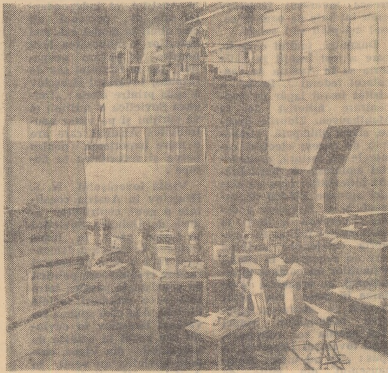
Iată în fotografia alăturată o vedere a Ciclotronului de la Institutul de Fizică Atomică al Academiei R.P.R.
