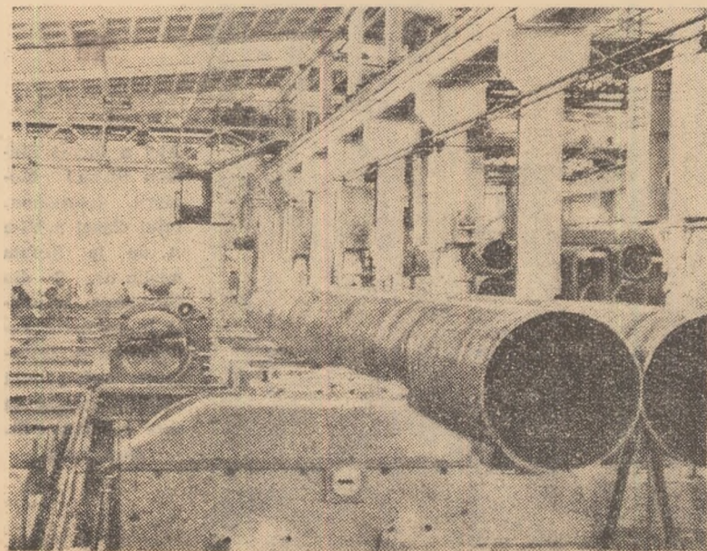
Aspect de la fabrica de țevi sudate-București.
